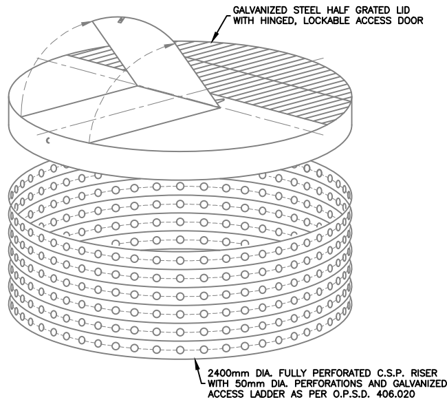
RISER PIPE LID DETAIL
